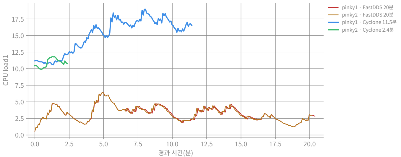
CPU load1 추이 (장시간 테스트)
