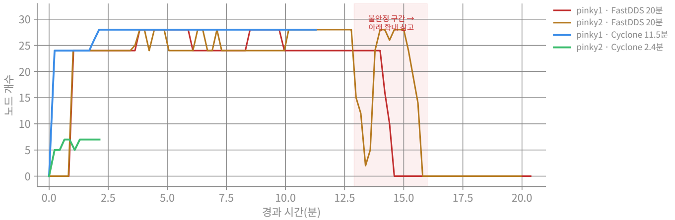
노드 디스커버리 추이 (전체)
